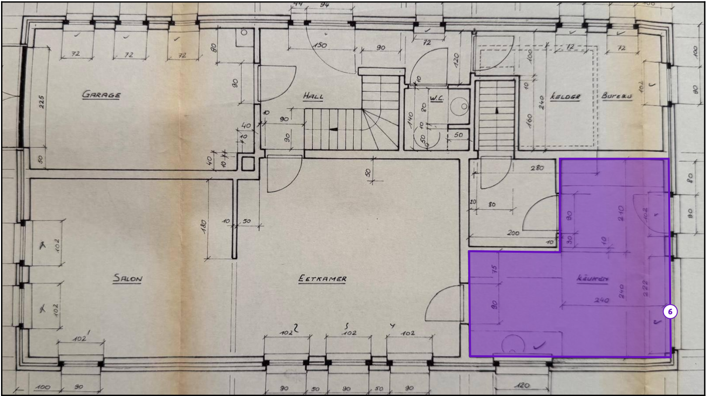
Legende van plan 1.3: Plafond plaat - gelijkvloers
