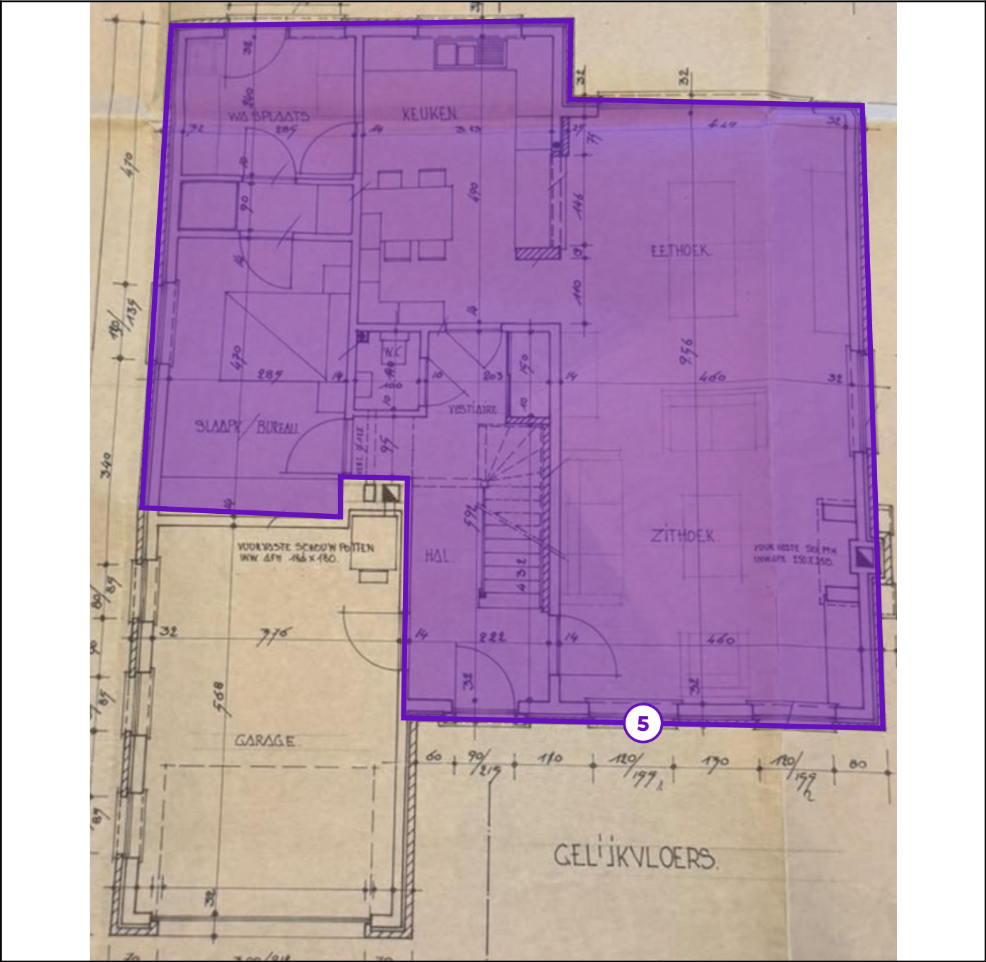
Legende van plan 1.3: Plafond plaat - gelijkvloers
