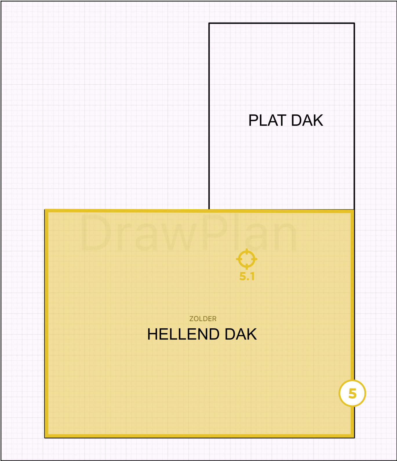
Legende van plan 1.8: Dakenplan - onderdak
