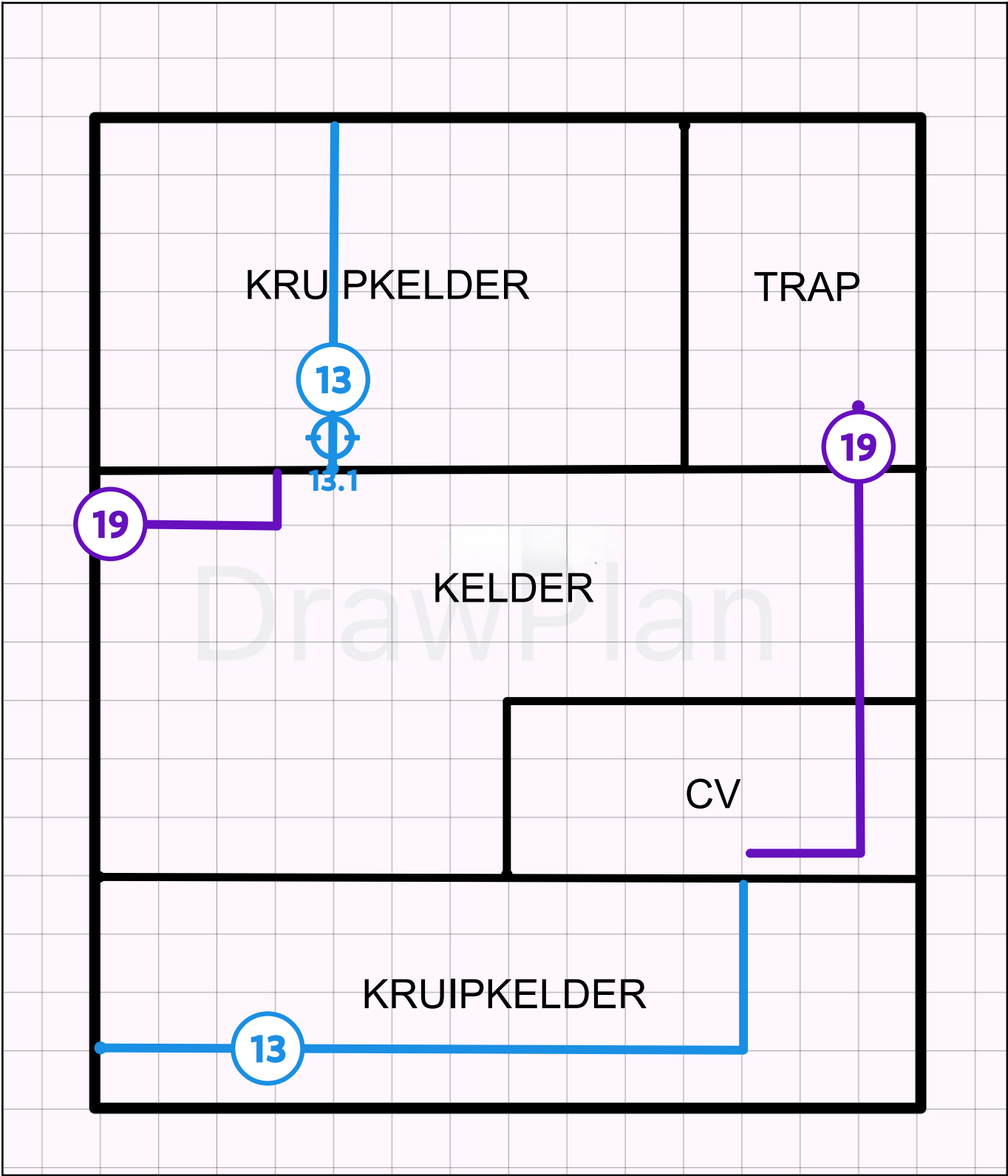
Legende van plan 1.13: Kelder - leidingsisolatie
