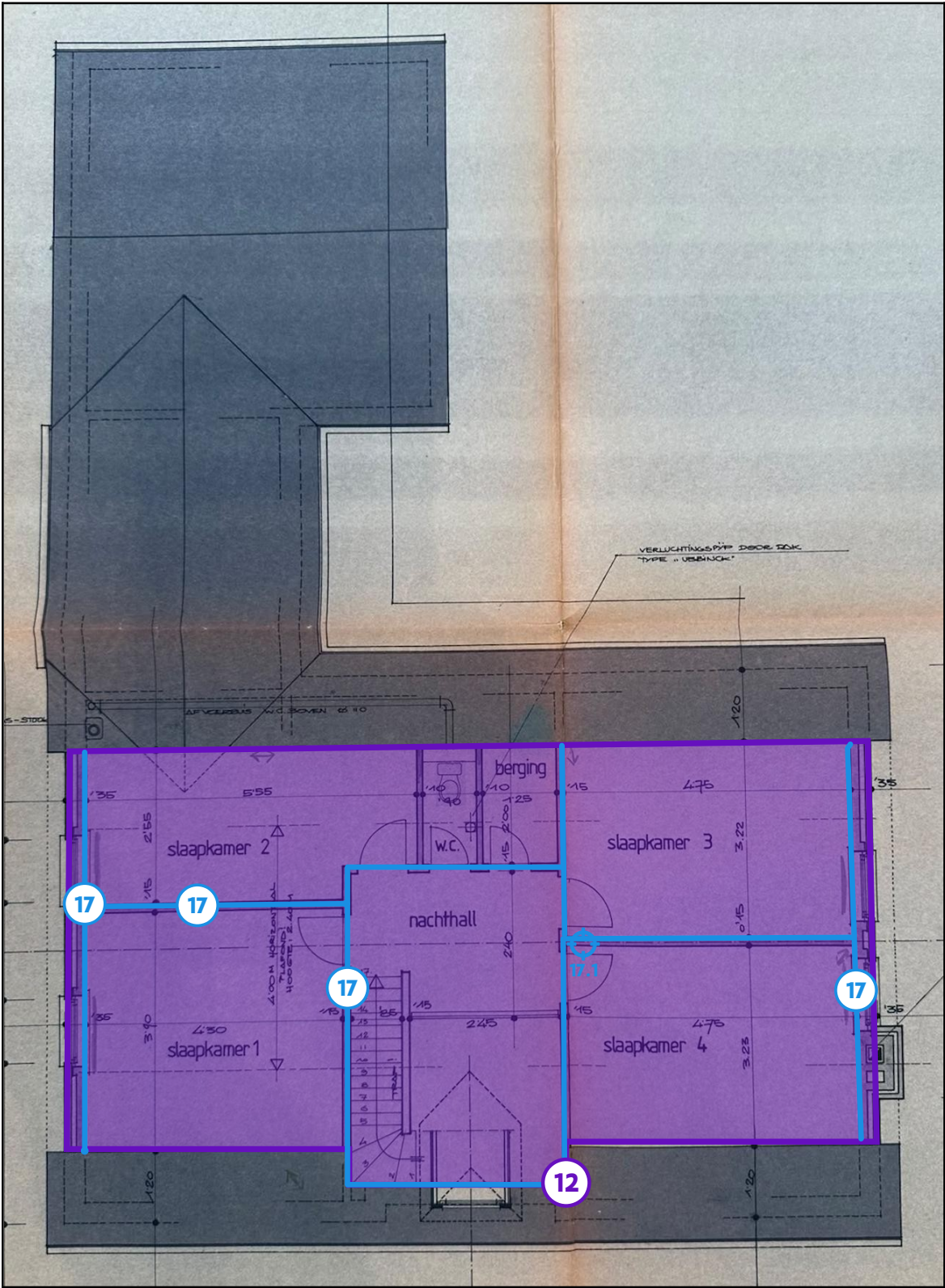
Legende van plan 1.6: Bezetting muur - plafond plaat eerste verdieping
